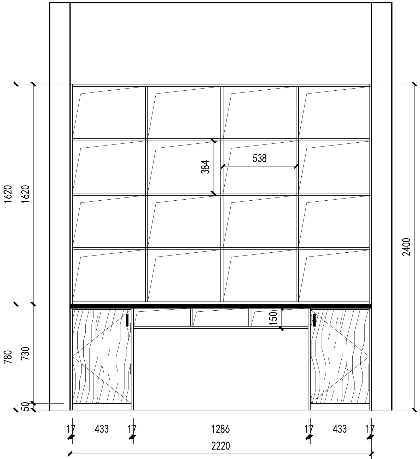
办公桌正立面图
